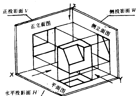
三面正投影图的形成
