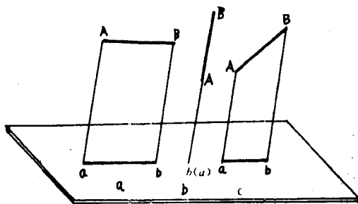
直线的投影
