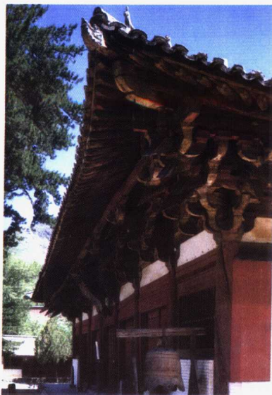
6-1 五台山佛光寺东大殿近景（唐代）
