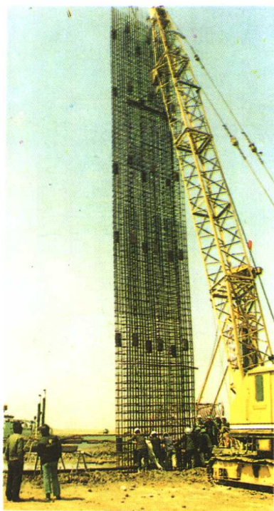
吊装钢筋笼子下槽
