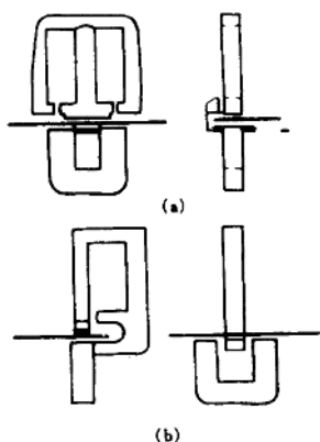
图 2-1 电磁元件 (a) 切线式；(b) 辐射式
