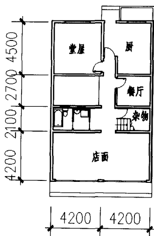
一层平面图
