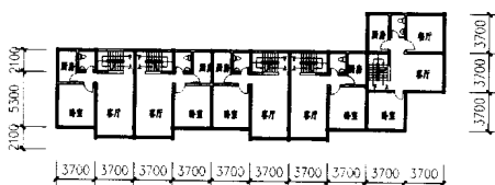
五层平面图
