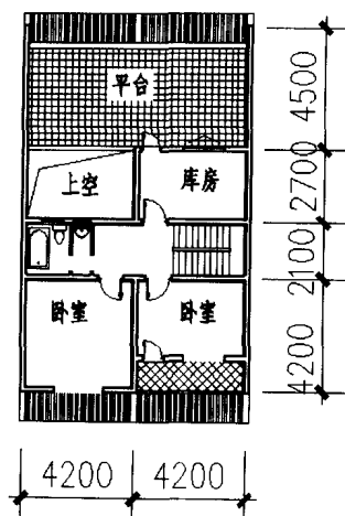
二层平面图
