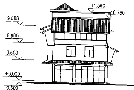
正立面图
