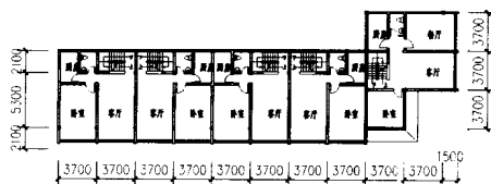
底层平面图
