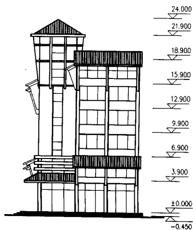
侧立面图
