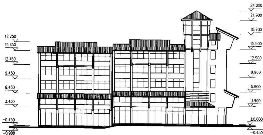
正立面图
