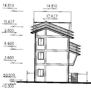
侧立面图
