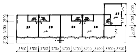
底层平面图
