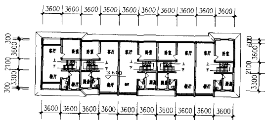
二层平面图
