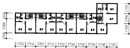
三、四层平面图
