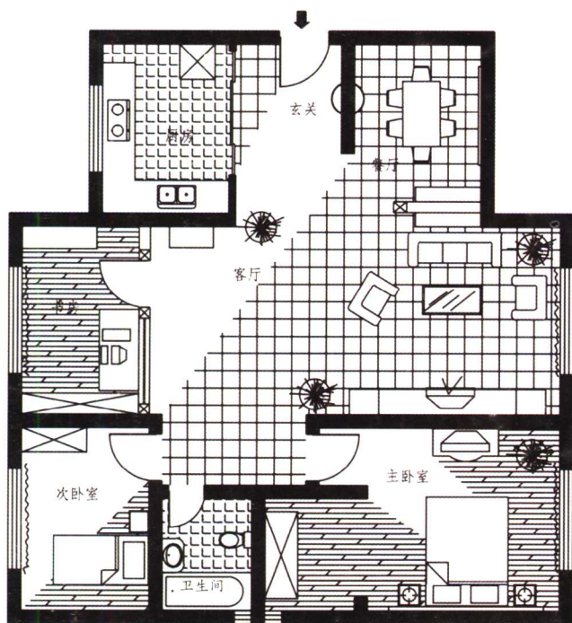
家庭装修平面布置图
