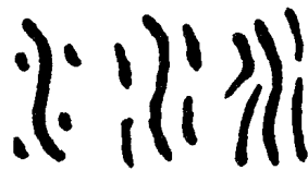
汉字的特殊形貌和构成 汉字是方块字。每个汉字在纸面上都占有一个方形的空间。
