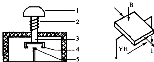
1.键帽 2.复位弹簧 3.键杆 4.磁钢 5.霍尔器件
