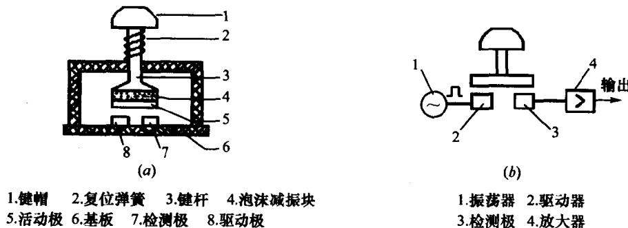
图 1-3 电容式键开关的结构和原理
