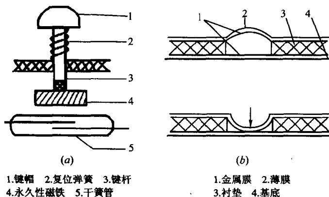
图 1-2 干簧管式和薄膜式键开关
