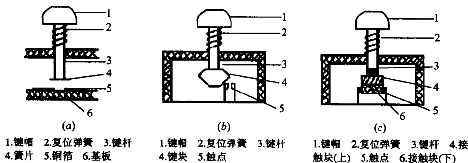
图 1-1 机械簧片式键开关 (a) 簧片式；(b) 触点式；(c) 导电橡胶式。
