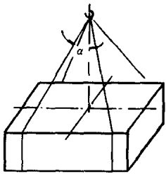
图 1-4 计算千斤绳拉力图示
