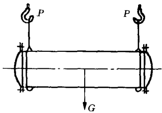
图 1-5 起吊水箱
