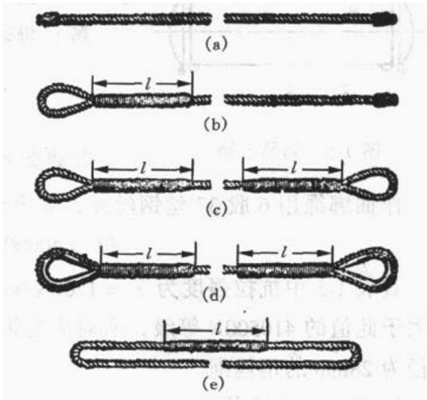
图 1-7 绳索
