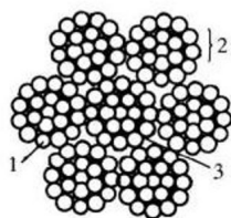
图 1-2 钢丝绳的断面
