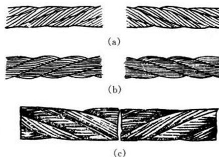
图 1-3 钢丝和股的绕捻方向
