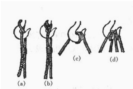
图 1-6 绳索缠勾法
