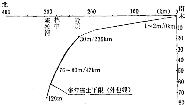
图 1—2 大小兴安岭多年冻土剖面分布规律示意图
