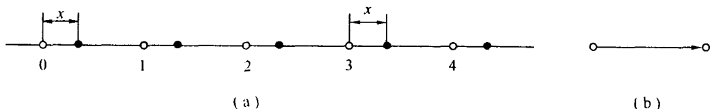
图 1-5 一维布喇菲格子
