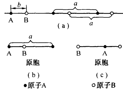
图 1-6 一维复式格子
