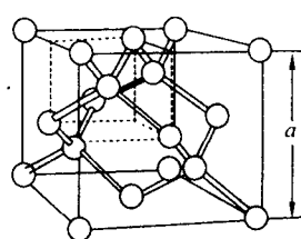
图 1-12 金刚石结构
