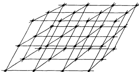
图 1-4 晶体的网格
