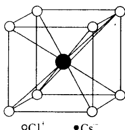
图 1-11 氯化铯结构
