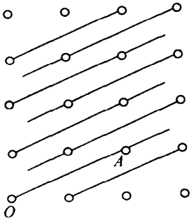
图 1-14 晶列
