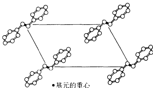
图 1-3 结点示意图
