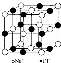
图 1-10 氯化钠结构
