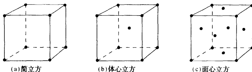
图 1-8 立方晶系布喇非原胞
