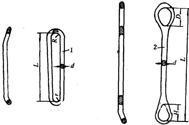
图 2-2 吊环结构
