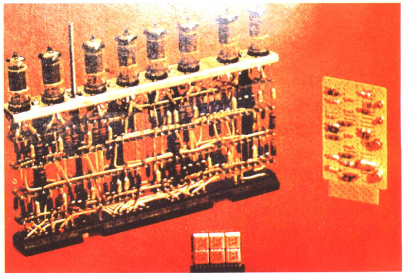
图 31 三代电子计算机零件
