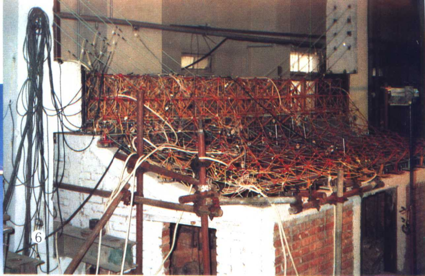
6 国家奥林匹克体育中心体育馆斜拉索双层网壳结构试验模型
