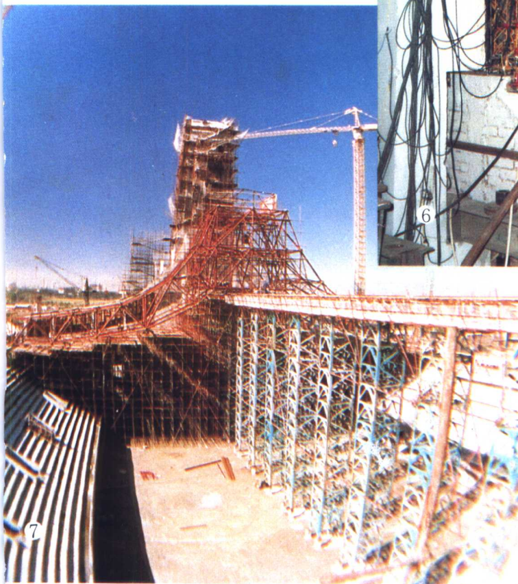
6 国家奥林匹克体育中心体育馆斜拉索双层网壳结构试验模型
