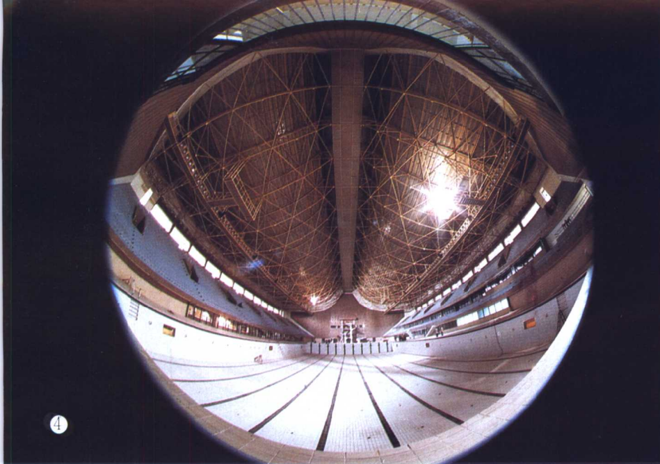
4 国家奥林匹克体育中心游泳馆斜拉索空间组合桁架
