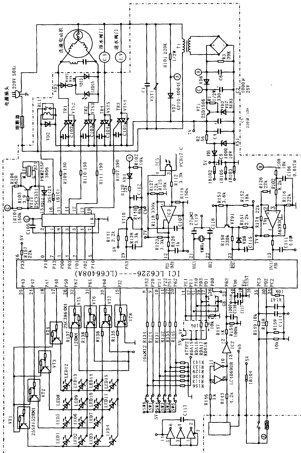
3. 三洋XQB50—68型洗衣机电气原理图
