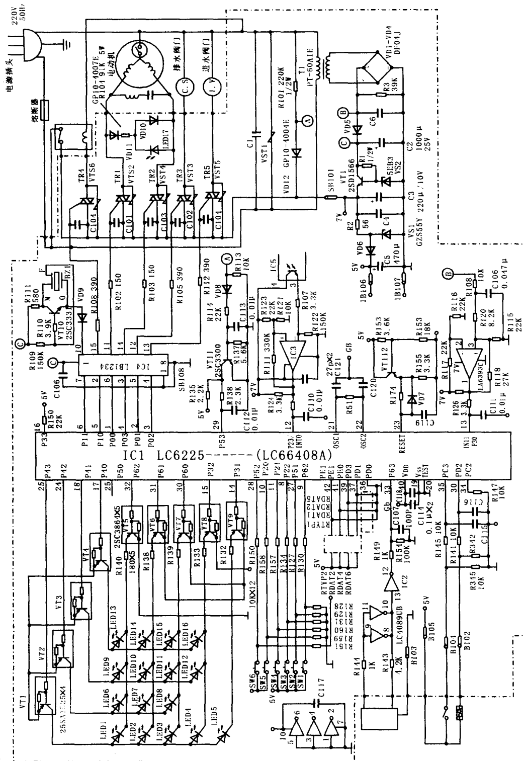
4. 三洋XQB50-168型洗衣机电气原理图
