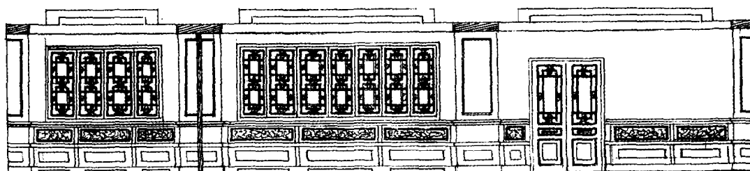
南立面图 1:50
