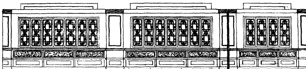
北立面图 1:50
