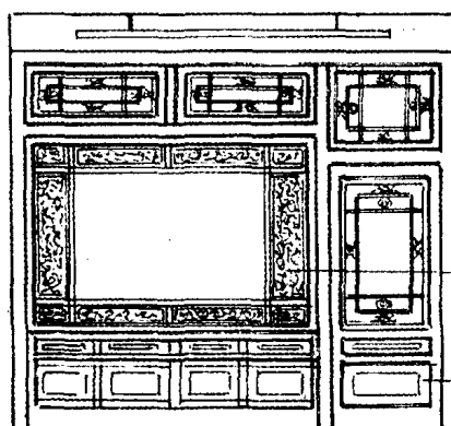
东立面 1:50
