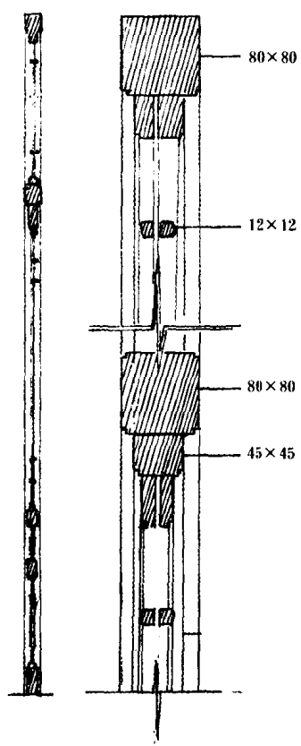
客厅结点图
