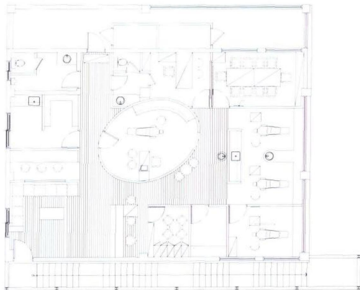
平面图
