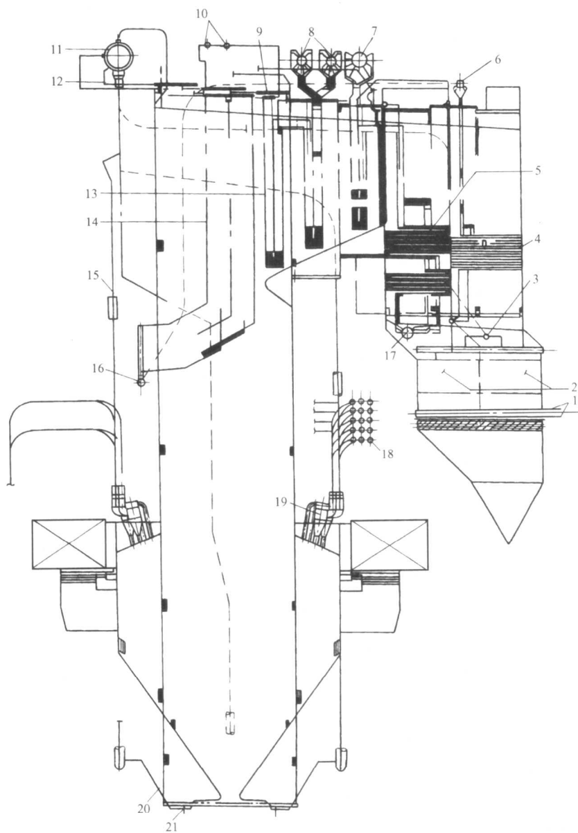
图 1-7 FW660MW 级 W 型火焰锅炉
