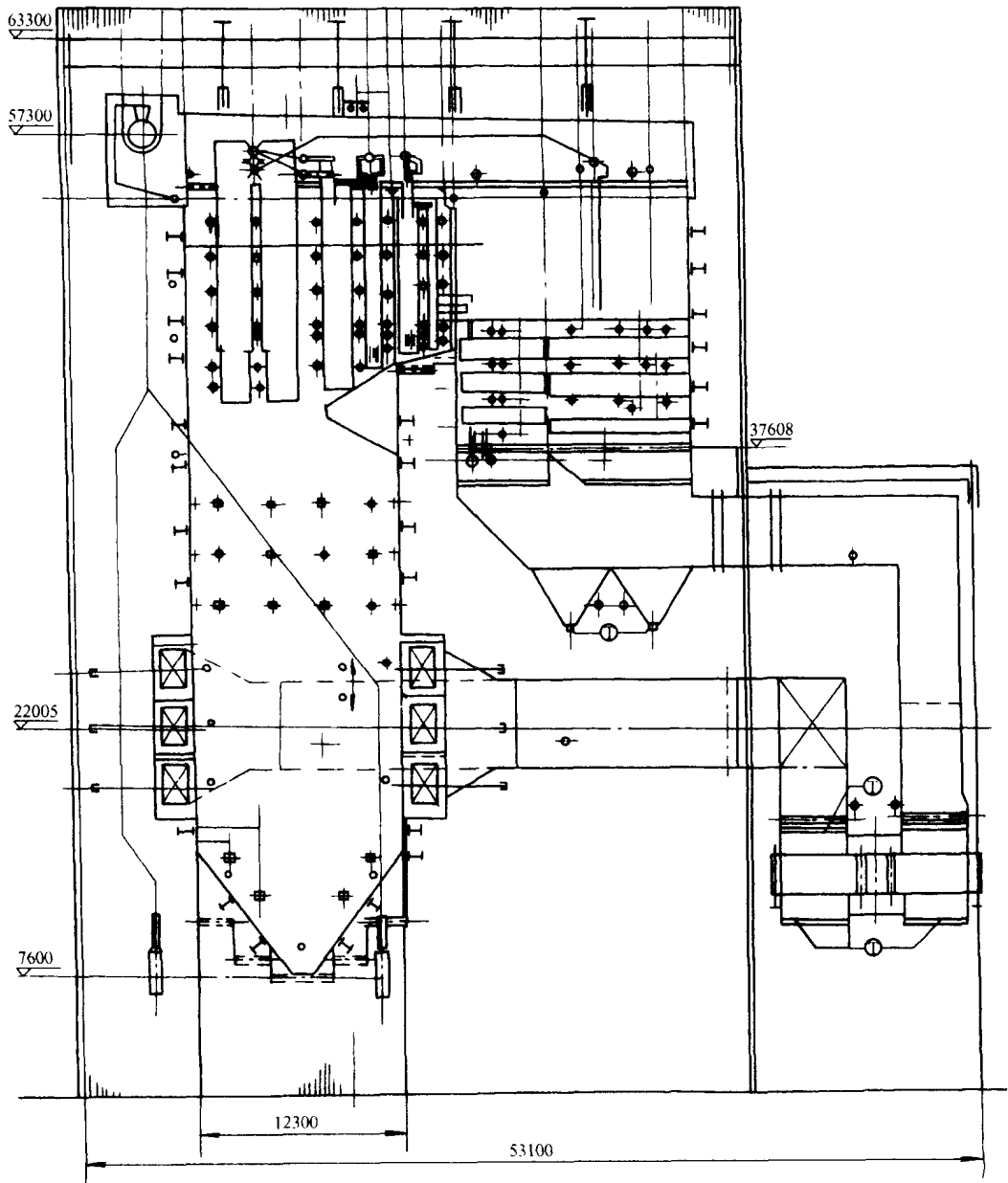
图 1-4 采用对冲燃烧的 300MW 锅炉
