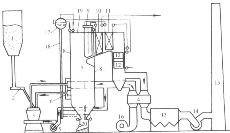
图 1-1 锅炉机组的工作过程示意
