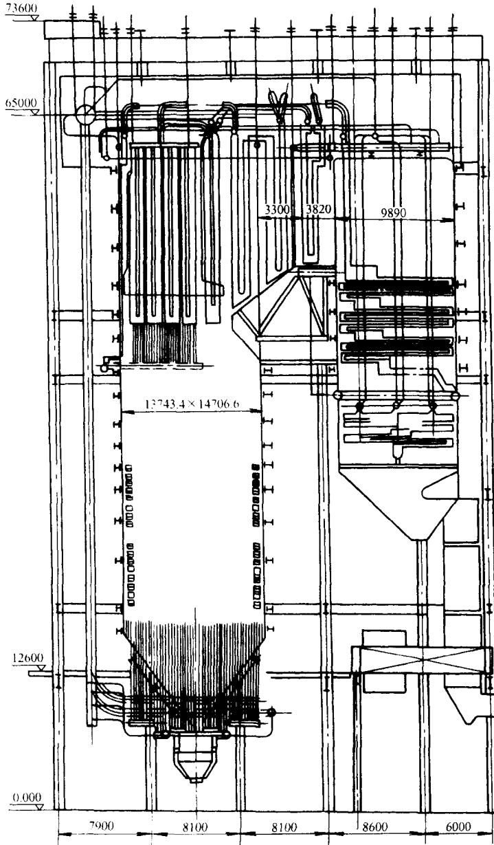
图 1-5 采用四角燃烧的 300MW 自然循环锅炉
