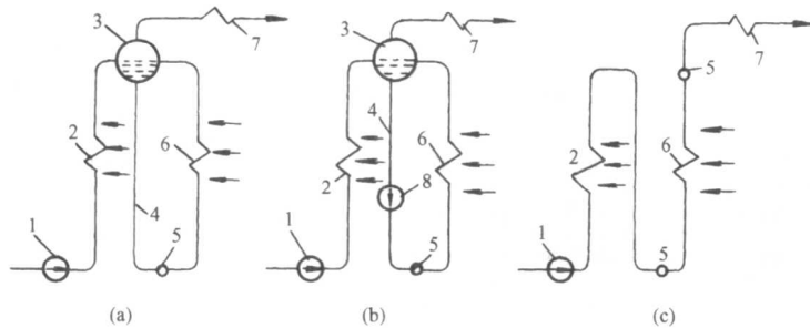
图 1-2 蒸汽锅炉蒸发部分的几种类型
