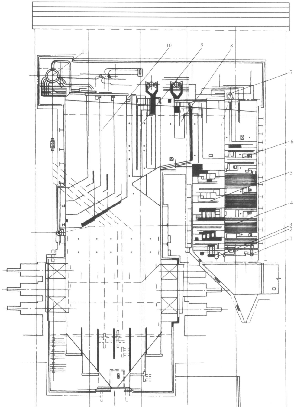
图 1-6 亚临界压力 600MW 自然循环锅炉
