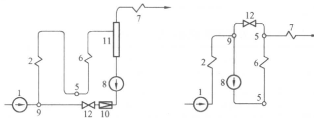
图 1-3 低倍率及复合循环系统
