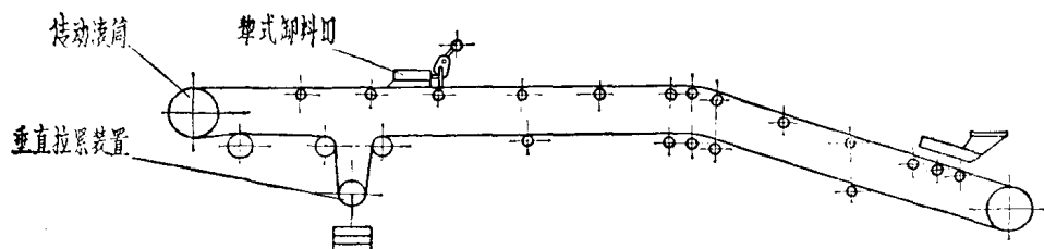
图2 装有垂直拉紧装置及犁式卸料装置输送机简图
