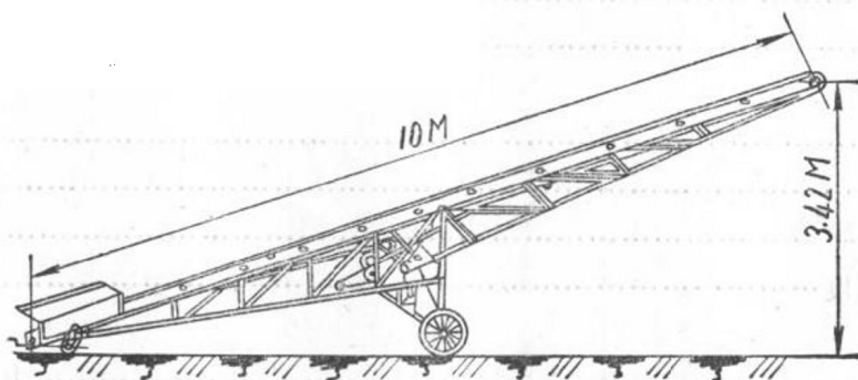
外形尺寸图
