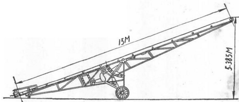
外形尺寸图
