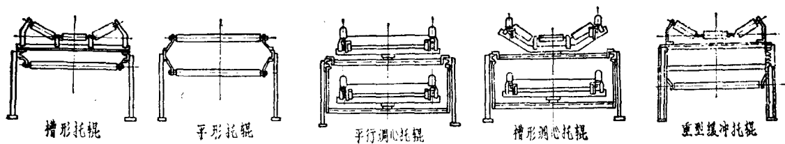
图1 带式输送机横断面图
