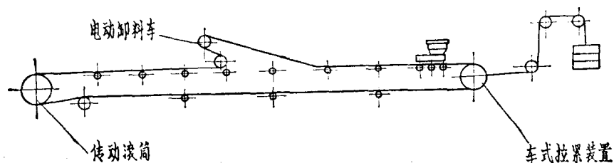
图3 装有车式拉紧装置及电动卸料车输送机简图
