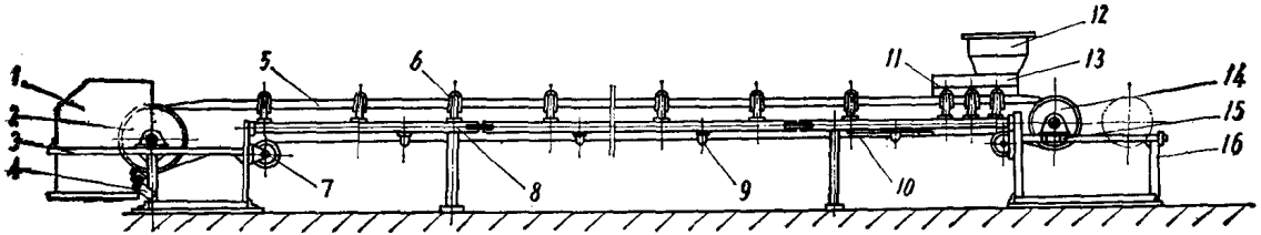
外形图
