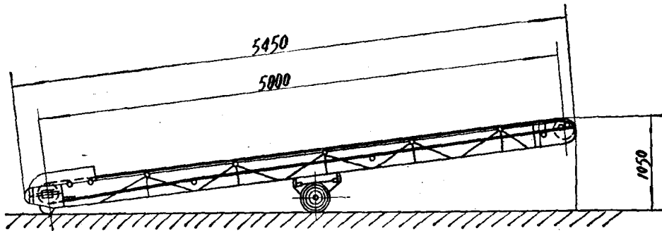
外形尺寸图
