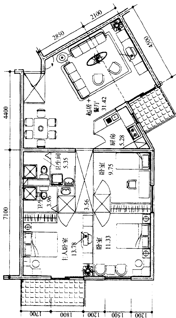
图 1-4 三室一厅设计方案(建筑面积 112.81 米 2 )
