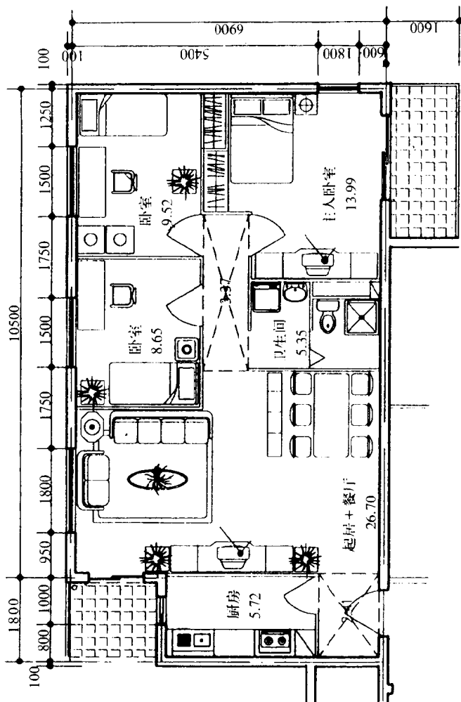
图 1-1 三室一厅的设计方案 (建筑面积 98.72 米 2 )
