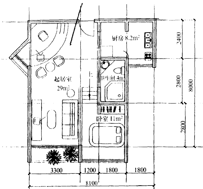
图 1-3 一室一厅夫妇居室设计方案(建筑面积 63.2 米 2 )
