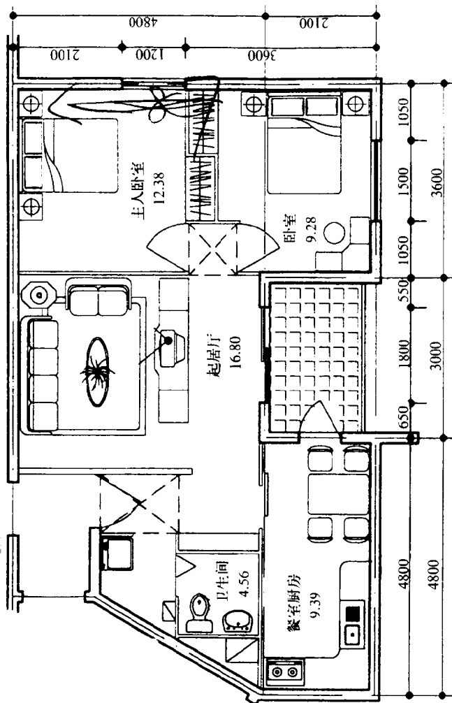
图 1-2 二室一厅的设计方案(建筑面积 73.83 米 2 )
