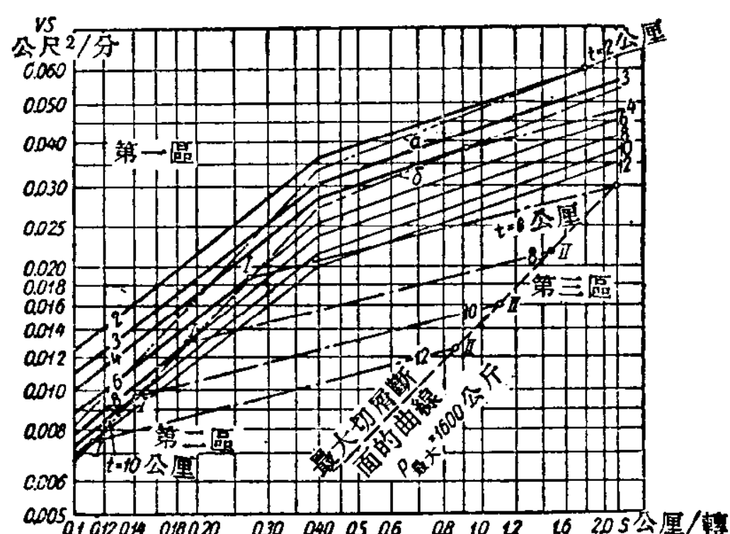
圖 1 [紅色無產者]工廠出品的 1Д62(ДИП-20) 型車床的生產特性:
