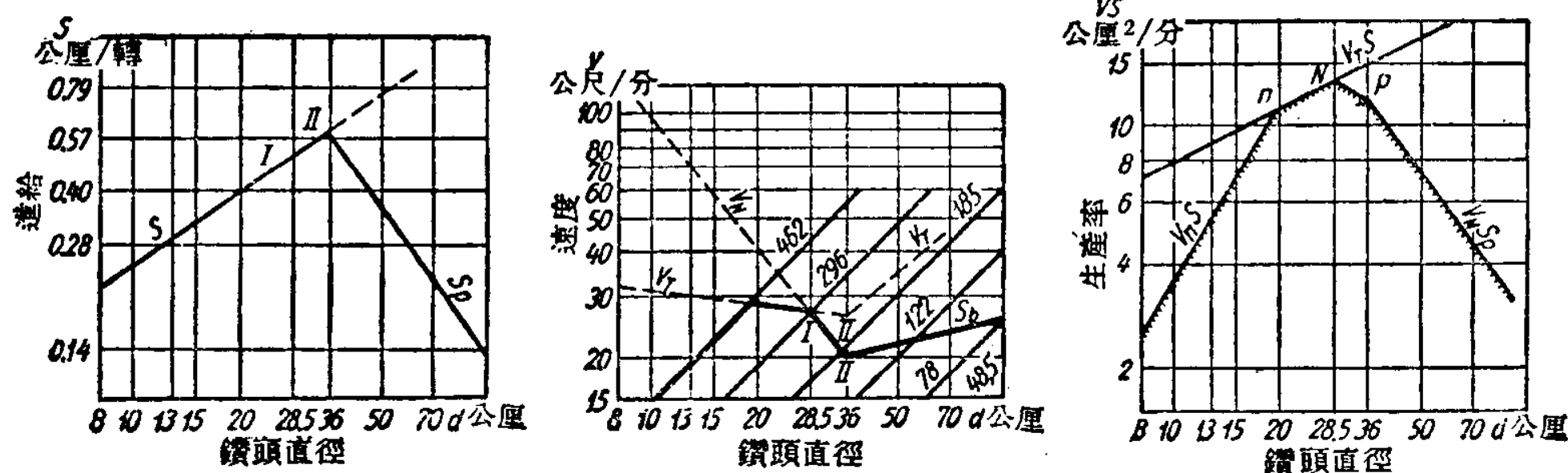
圖 2 2135 型立式鑽床的生產特性。
