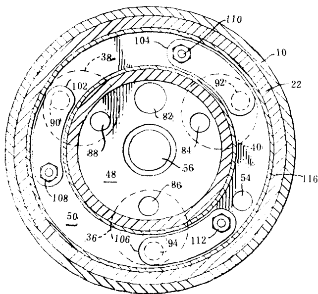
图 2-3 I-I 剖视
