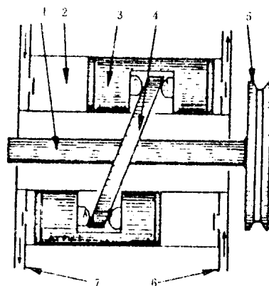
图 2-1 斜盘压缩机示意图
