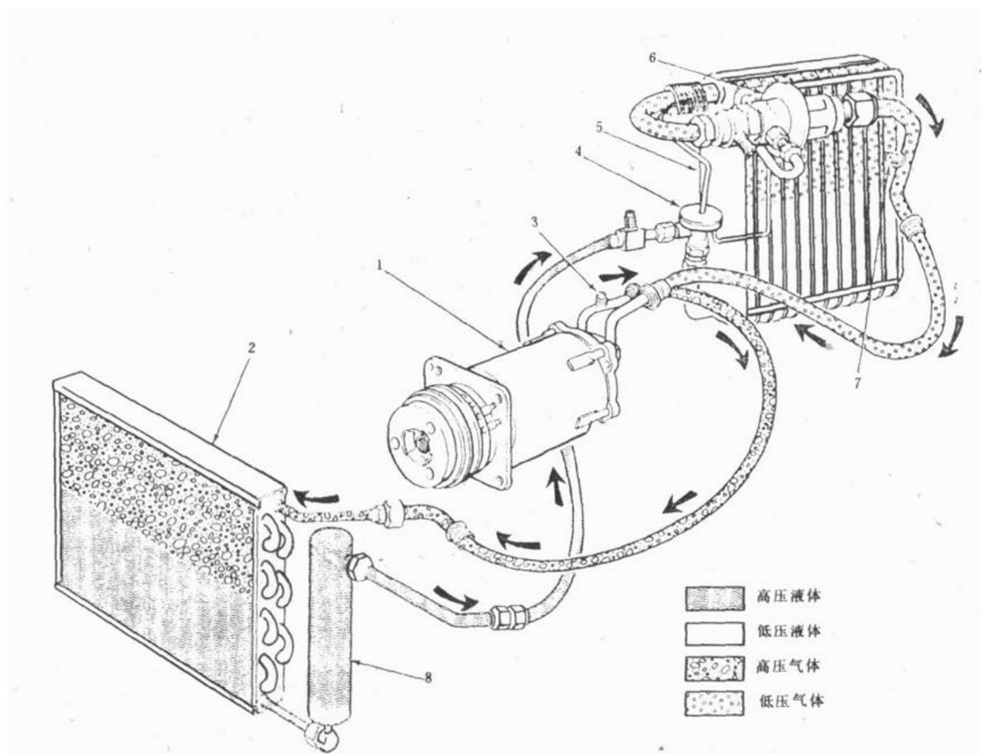
图 1-4 汽车空调系统
