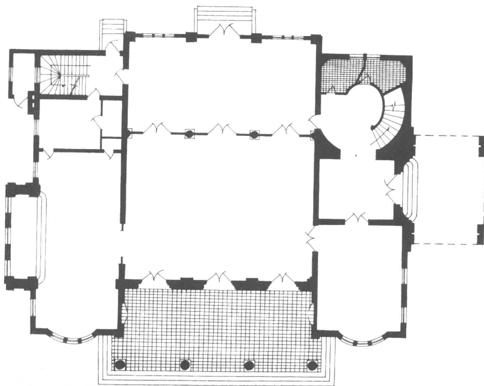
一层平面图
