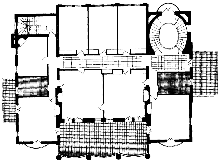
二层平面图
