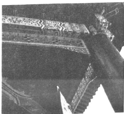
图15 清·颐和园德和园大戏楼(中) 及寿台之仙楼(上)、天井(下)
