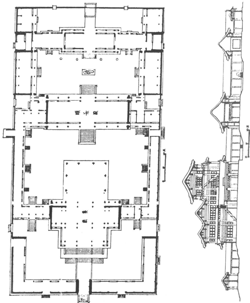
图 16 颐和园德和园大戏楼平面及剖面图
