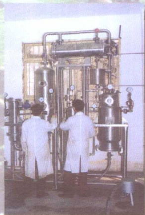
药物研究所多功能提取罐
