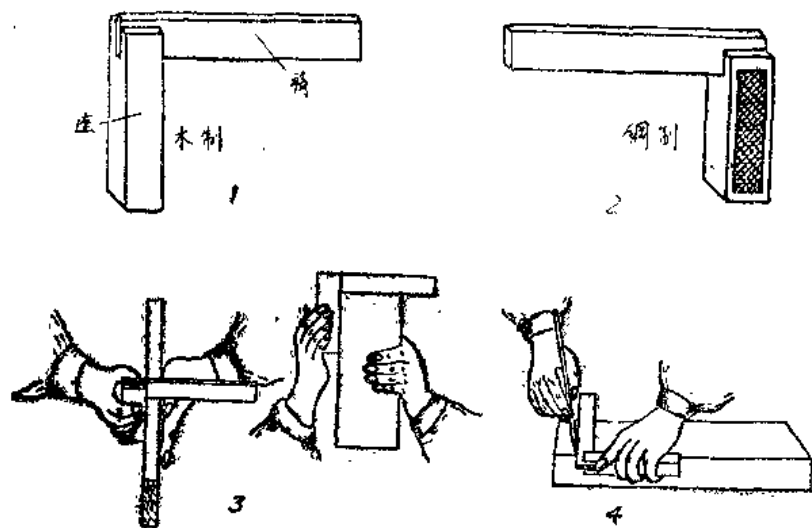
图4. 直角尺形状及用法：
