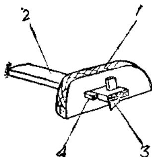
图13. 單綫勒子： 1—勒子擋；2—勒子杆； 3—小刀片；4—活楔。
