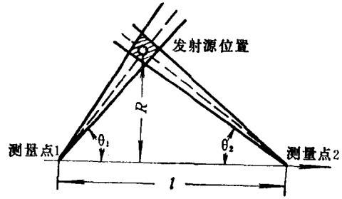
三角测量定位法示意图
