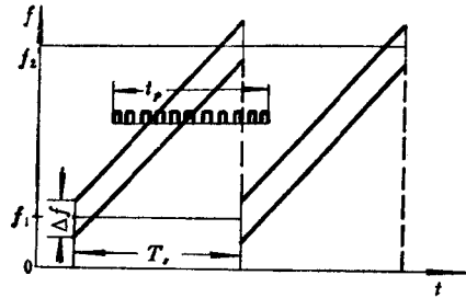
单程搜索测频的频率-时间图
