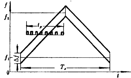
双程搜索测频的频率-时间图
