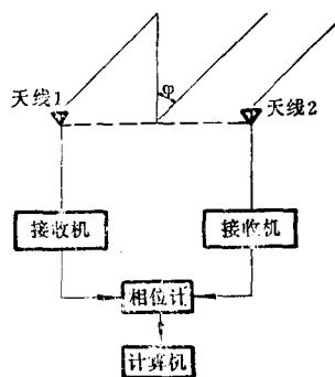
函数测向(相位比较)系统示意图
