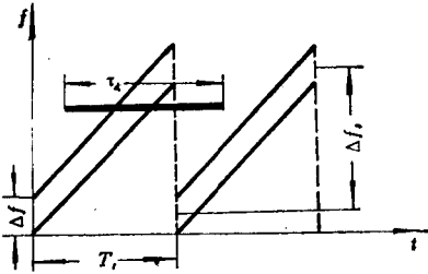
快搜索的频率-时间图
