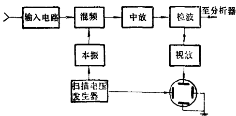
搜索接收机方框图
