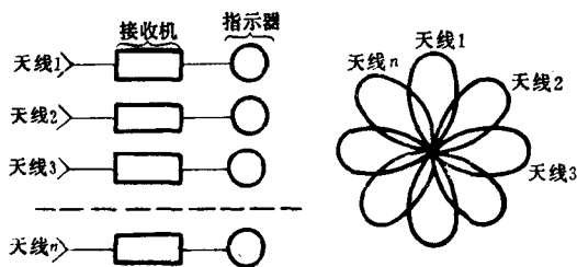
一种非搜索测向系统示意图
