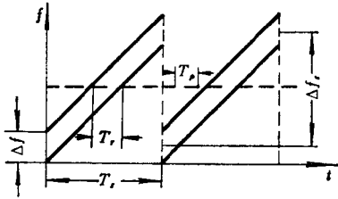
慢搜索的频率-时间图
