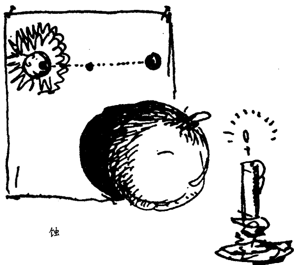
只有圆形物体才有圆形投影
