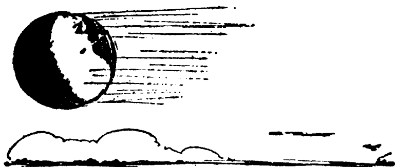
地球在宇宙中运行的速度比最快的炮弹快得多
