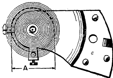
圖 1-11 游絲的直徑
