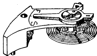
圖 1-4 裝置挑匡游絲的擺輪上夾板
