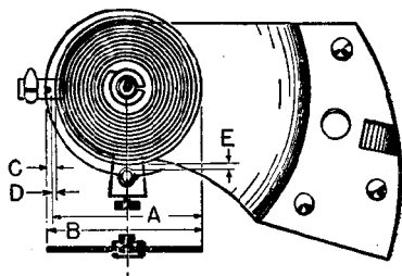
圖 1-12 游絲裝在擺輪上夾板上
