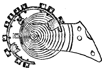
圖 1-7 游絲直徑過大
