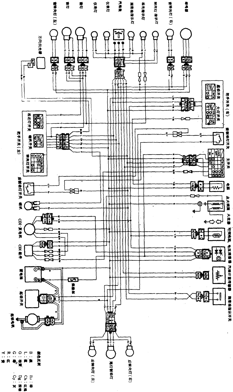
雅马哈 CR50 型踏板式两轮摩托车电路图
