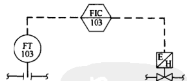
图 30-3 计算机控制（无后备，集中指示）
