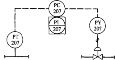
图 30-11 模拟控制（无显示调节器、集中显示）
