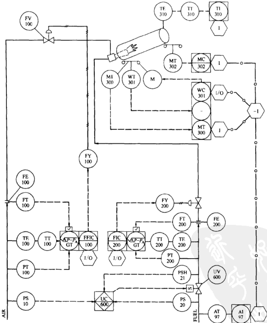
图 30-16 流程简化图示例
