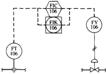
图 30-6 计算机控制（从集散控制仪表开始全部后备，计算机使用仪表系统通讯总线）
