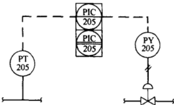
图 30-8 集中显示/分散控制（具有辅助操作员接口设备）
