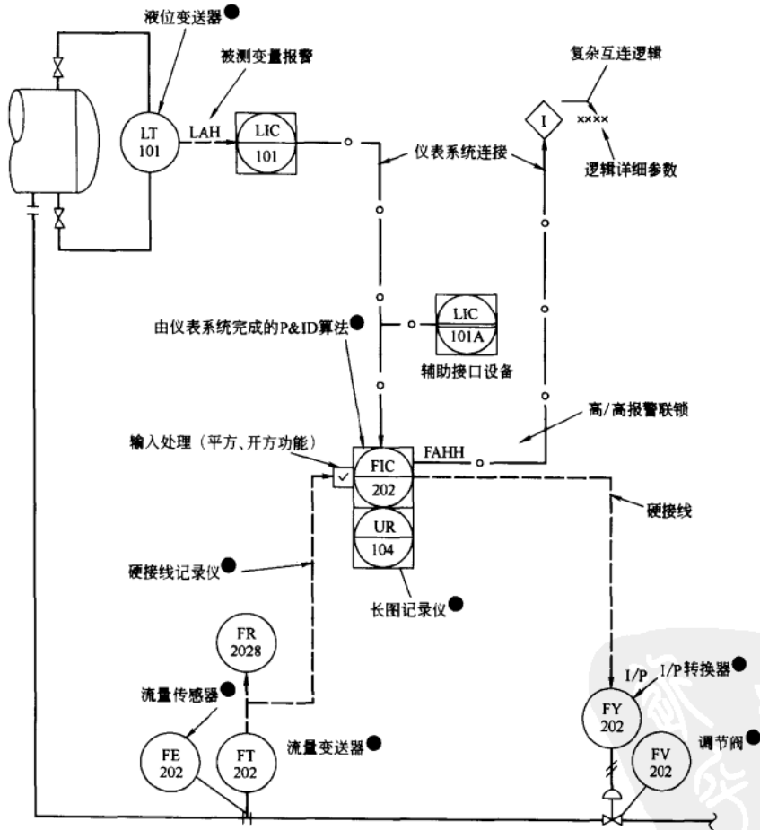
图 30-17 申级调节回路典型流程图
