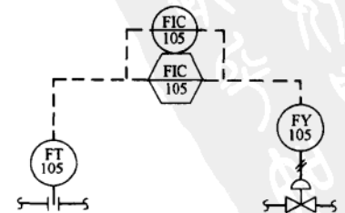
图 30-4 计算机控制（具有模拟后备）
