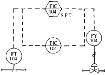
图 30-5 计算机控制（具有设定点跟踪 SPT 的全部模拟后备）
