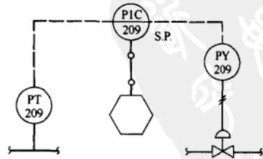
图 30-13 监督设定点控制（带常规面板的模拟调节器，通过通讯连接的计算机监督设定点）
