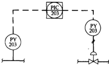
图 30-7 集中显示/分散控制（无后备）
