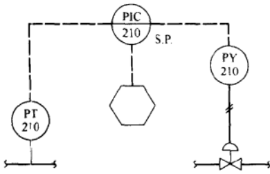
图 30-14 监督设定控制 (装备有常规面板的模拟调节器, 计算机监督设定点硬接线)
