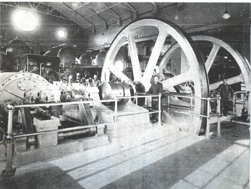
杨树浦水厂原9号蒸汽唧机
