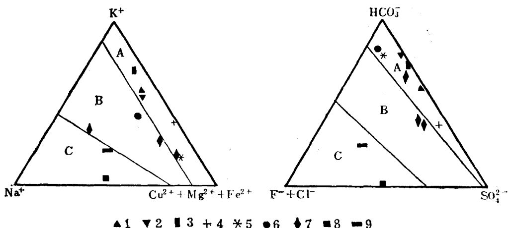
图 1 流体包裹体液相成分图解
