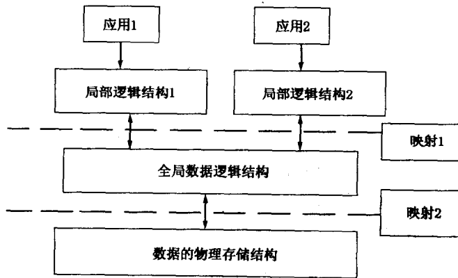
图 1-5 应用程序和数据库的映射
