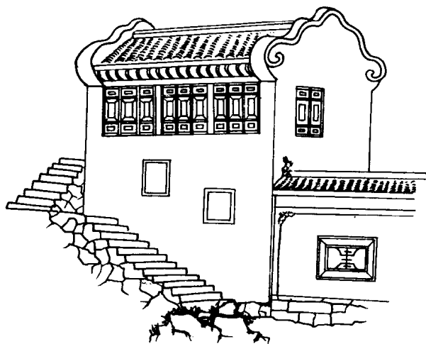
福建楼式住宅外观
