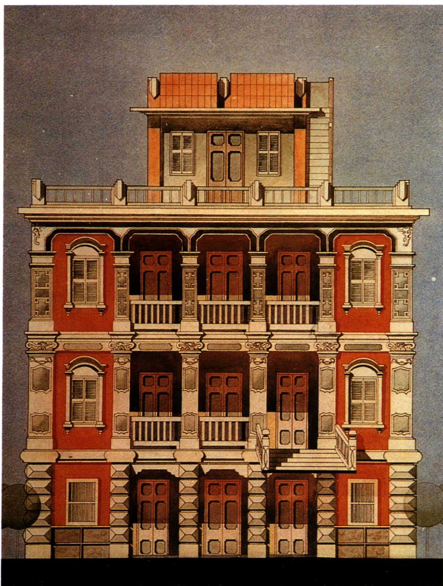
鼓浪屿宾馆（黄奕柱别墅）绘图：沈琼（天津大学建筑系）
