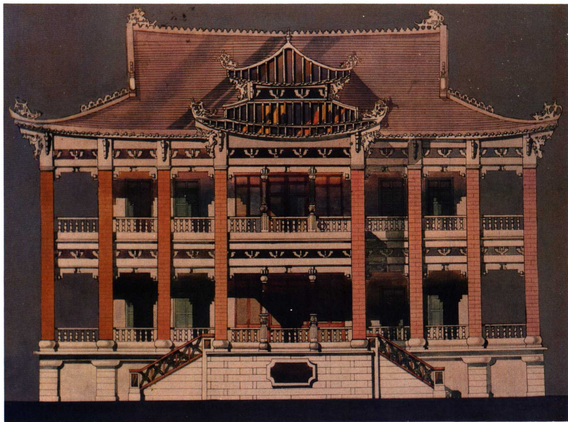
“海天堂构”正立面图 绘图：李学俊（天津市规划局）
