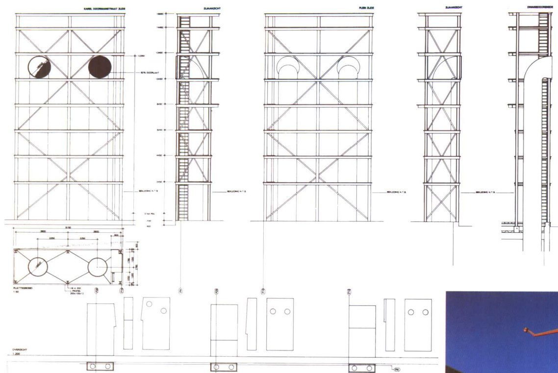
地下停车场通风井详图。
