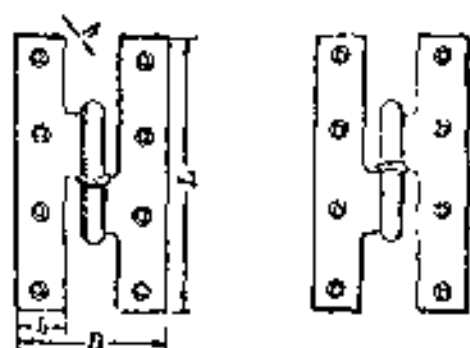
右铰
