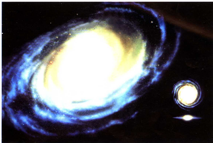
银河系全貌(银河系是典型的漩涡星系,直径达10万光年)
