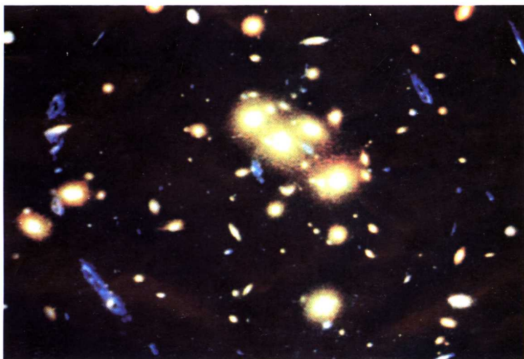
“哈勃”太空望远镜近期拍摄到的最遥远星系图像
