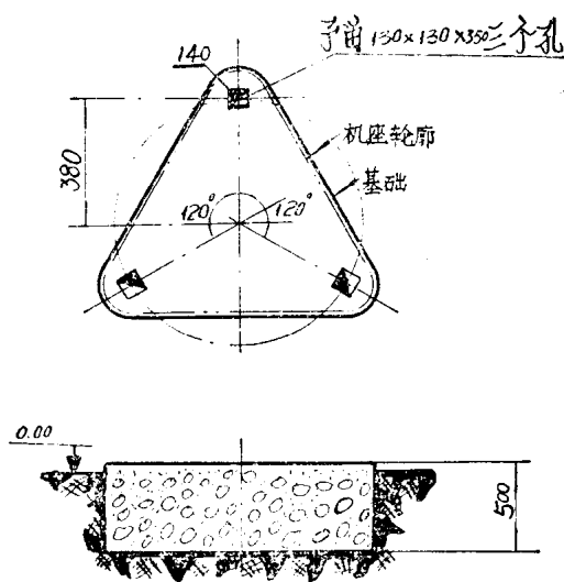
SS-450型离心机基础图
