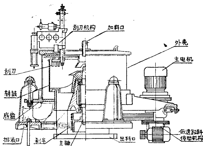
SX型三足式下部卸料离心机结构图
