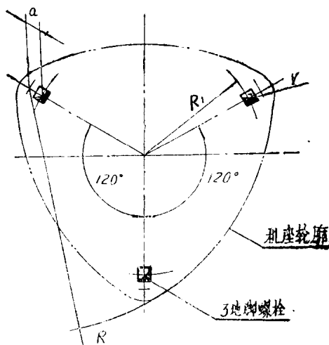
SS— 600 / 800 型离心机基础图
