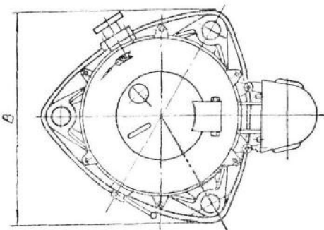
SS- 600 / 800 型离心机剖面和外形尺寸图
