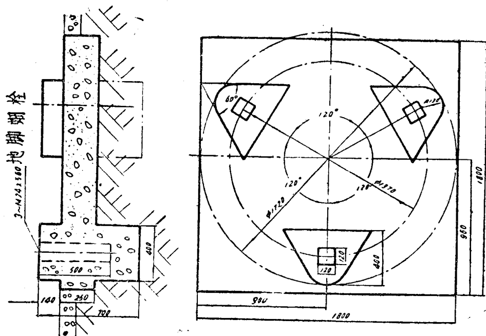
SS—1000型离心机基础图
