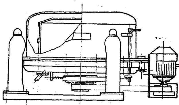
SS-450型离心机剖面图
