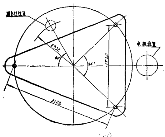
SS—1800型离心机基础图
