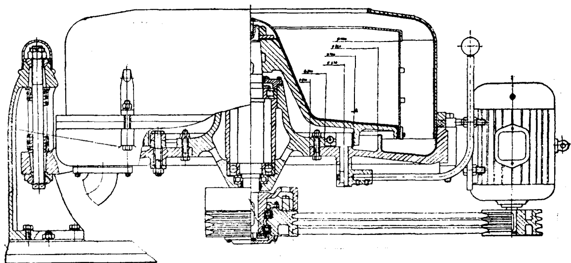
SS—1000型离心机剖面图
