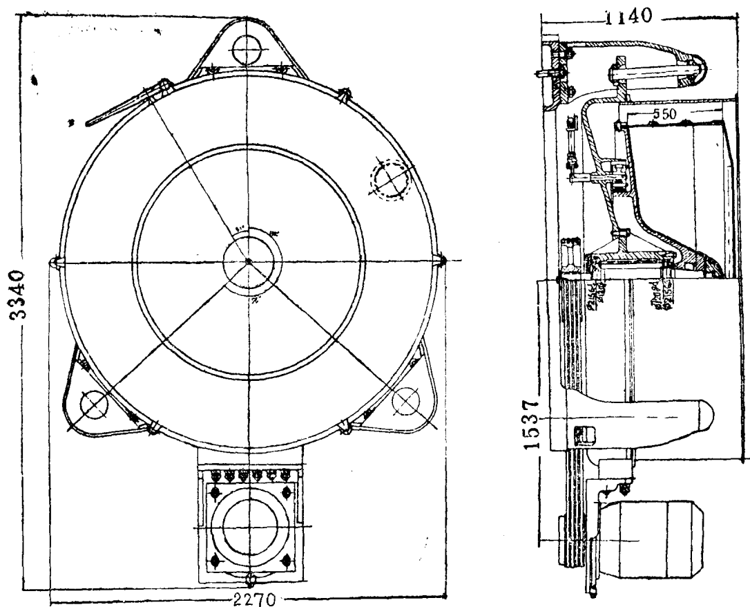
SS—1800型离心机剖面图
