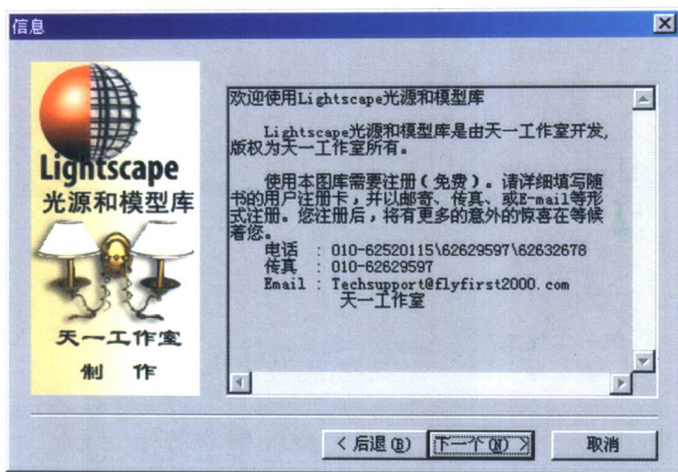
图4 信息窗口
