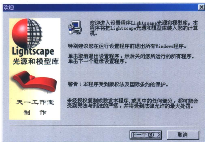
图 2 安装界面
