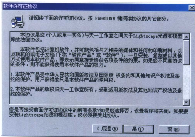
图 3 安装信息栏
