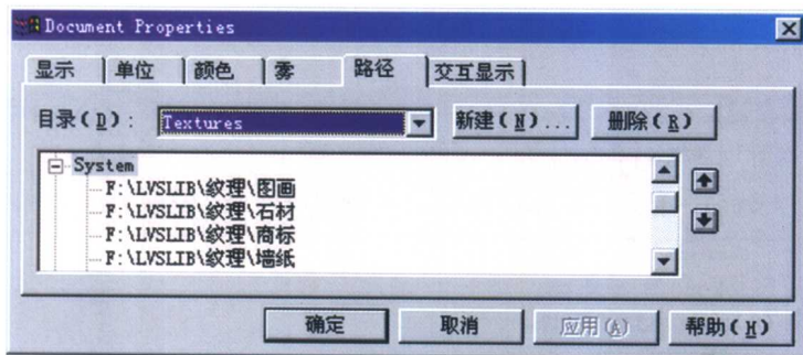
图 18 纹理路径 2
