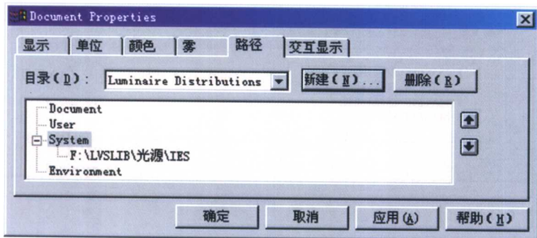
图 16 光域网路径
