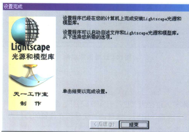
图13 设置完成
