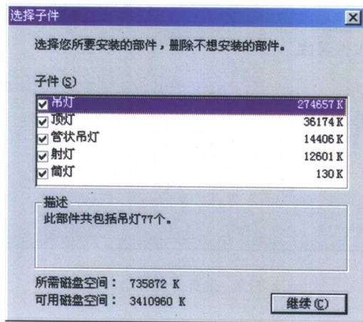
图11 选择子件
