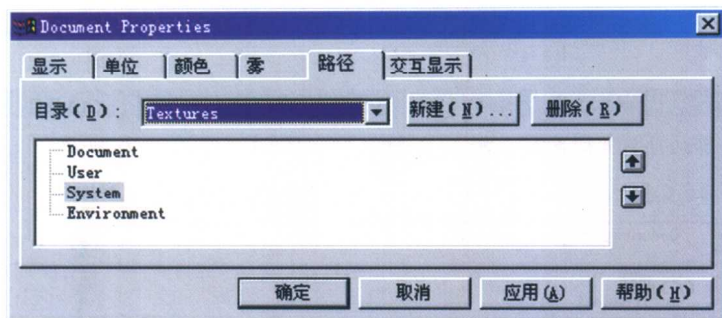
图 17 纹理路径 1
