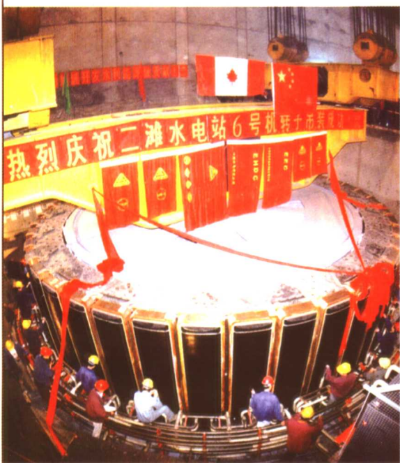
1998年2月25日首台机组转子吊装
