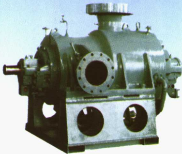
DAS系列双壳体多级中开泵
