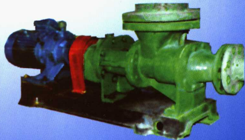
SB型双螺杆污泥泵
