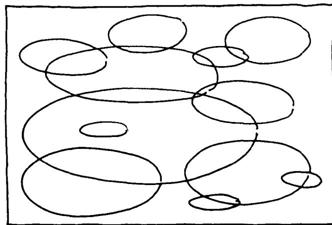
椭圆
