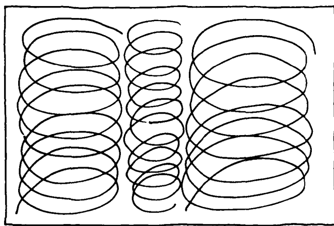
螺旋线
