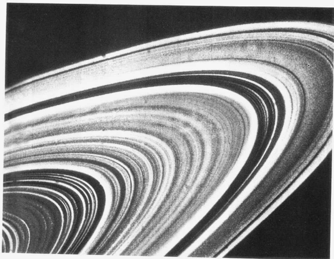
西姆斯第一个认为土星环就是土星存在空洞的证据。(上)
