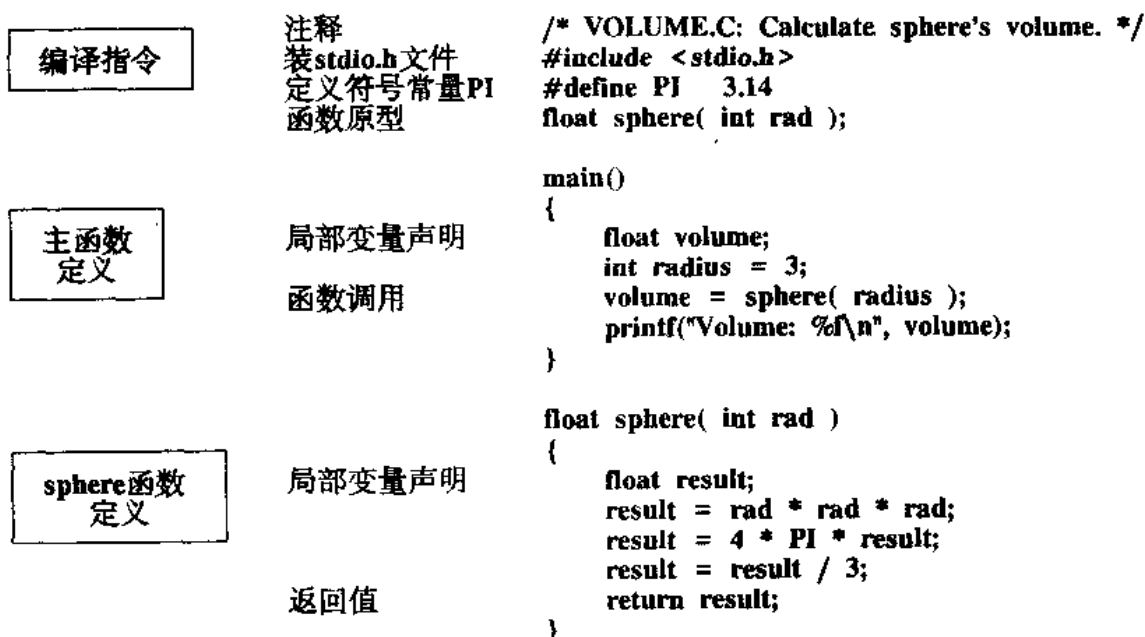
图 1.1 VOLUME.C 程序
