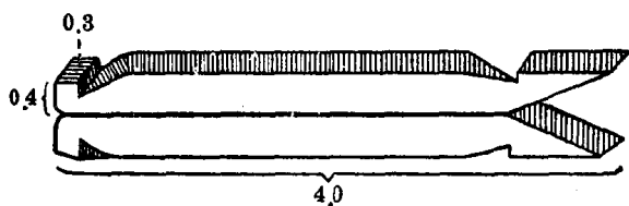
图 3 药割夹板(单位: 寸)
