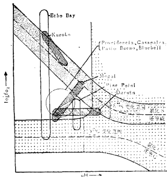
图 1 表示九个热液矿床恢复其沉积环境的 \text{pH}-f_{\text{O}_2} 图解 (引自Jensen and Bateman 1979)
