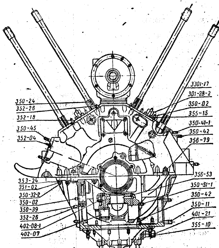
圖 6 曲軸箱。C6.301-15-12(机械部件)
