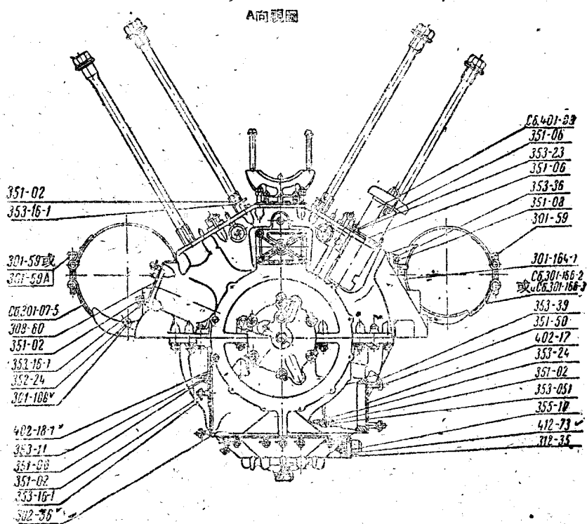
圖 4 曲軸
