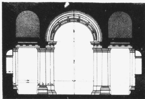
Coupe sur la largeur du vestibule d'entrée
